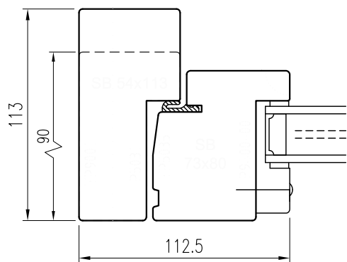
Horizontalsnitt
