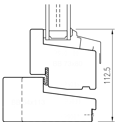
Vertikalsnitt EFU Öp
