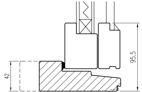
Fönsterdörr Tröskel
