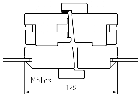
Vertikalsnitt KFU
