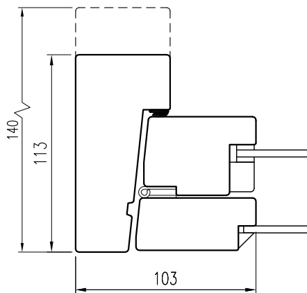
Horizontalsnitt KFU
