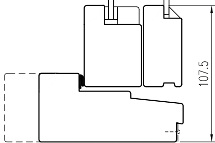
Vertikalsnitt KFU
