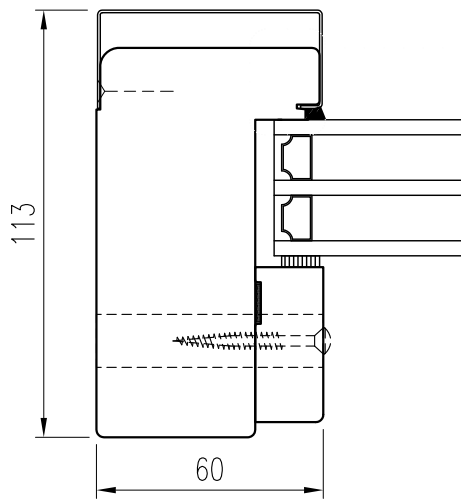
Horizontalsnitt
