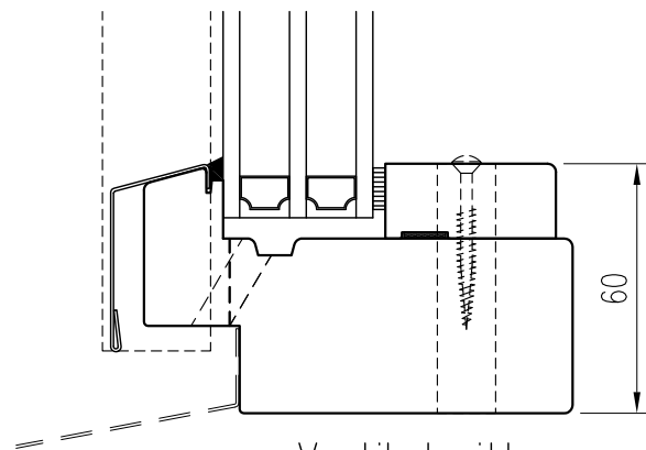
Vertikalsnitt
