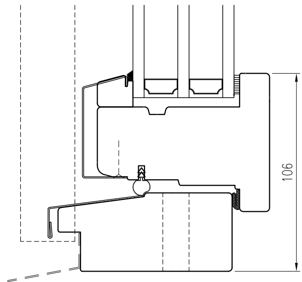
Vertikalsnitt
