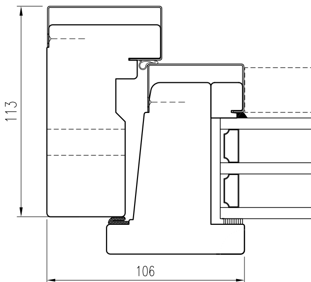
Horizontalsnitt
