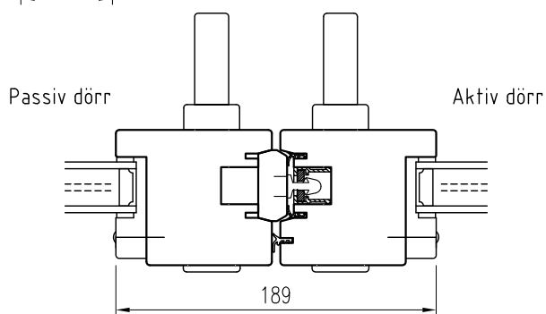
Horizontalsnitt pardörr
