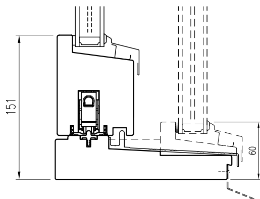
Vertikalsnitt med låg bottenbit i fast del Fast del ritad med streckad linje
