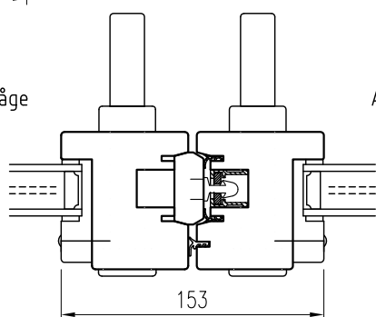
Horizontalsnitt pardörr/fönster
