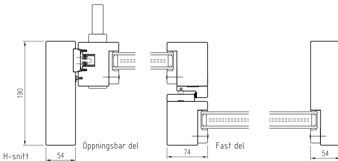
Passiv båge
