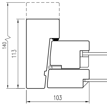
Horizontalsnitt KFU
