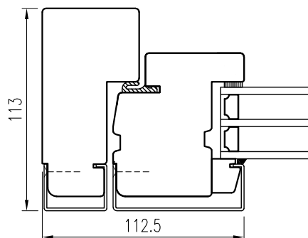
Horisontalsnitt
