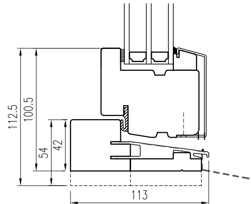
Vertikalsnitt Fönsterdörr
