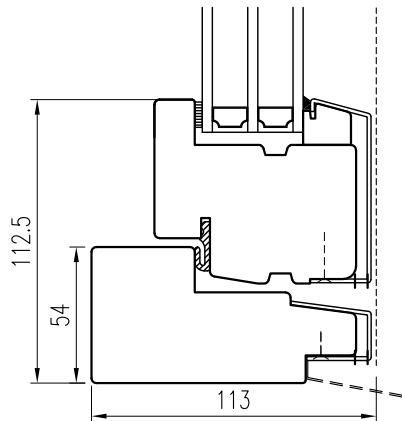
Vertikalsnitt Fönster
