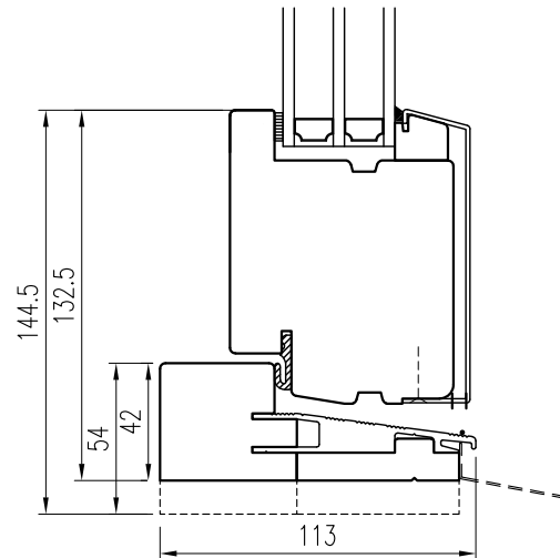
Vertikalsnitt
