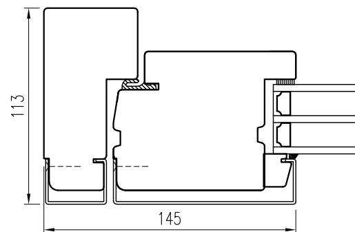
Horizontalsnitt
