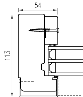
V-snitt glasning inifrån
