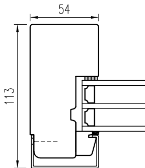
V-snitt glasning utifrån
