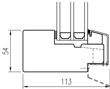
V-snitt glasning utifrån
