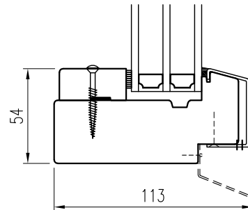
V-snitt glasning inifrån
