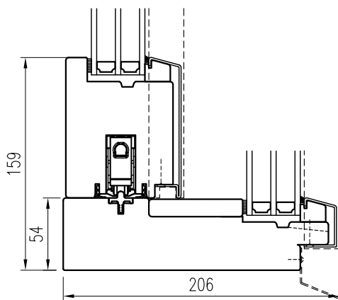
Vertikalsnitt med slimmad bottenbit i fast del
