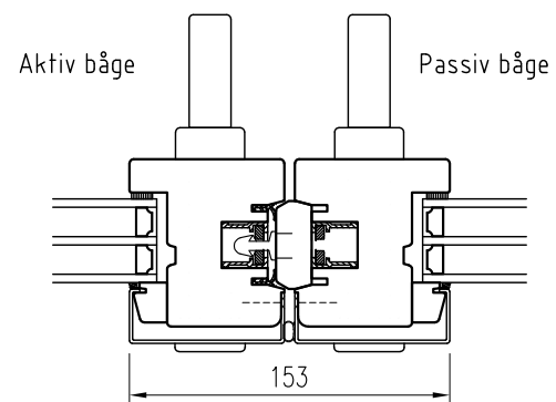
Horizontalsnitt pardörr Öppningsbar del
