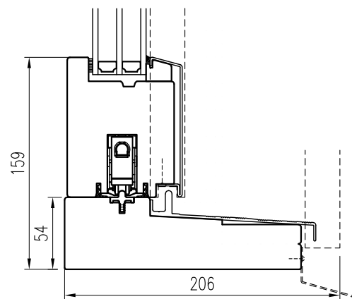
Vertikalsnitt öppningsbar del
