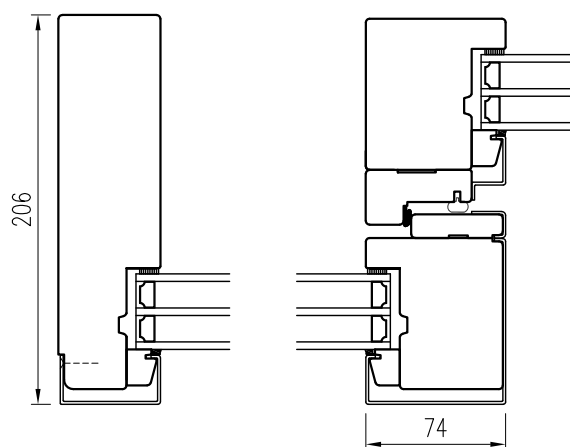
Horizontalsnitt pardörr Öppningsbar del
