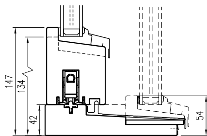
Vertikalsnitt 42mm tröskel med låg bottenbit i fast del Fast del ritad med streckad linje
