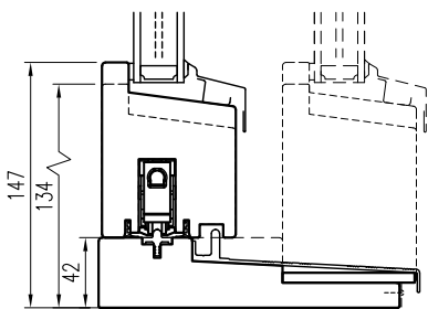
Vertikalsnitt 42mm tröskel med hög bottenbit i fast del Fast del ritad med streckad linje
