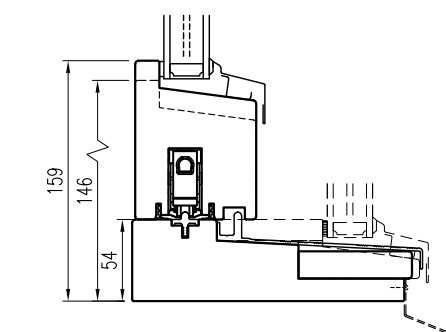
Vertikalsnitt 54mm slimmad tröskel Fast del ritad med streckad linje
