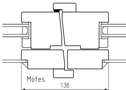
Fönsterdörr Tröskel
