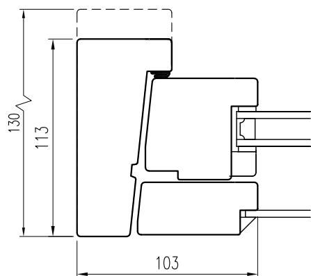
Horizontalsnitt KFU
