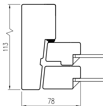
Horizontalsnitt KFU
