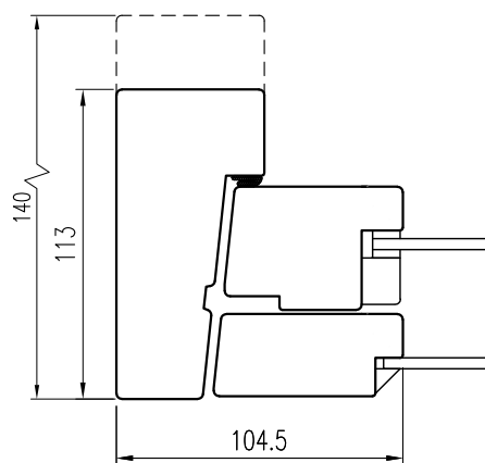
Horizontalsnitt KFU
